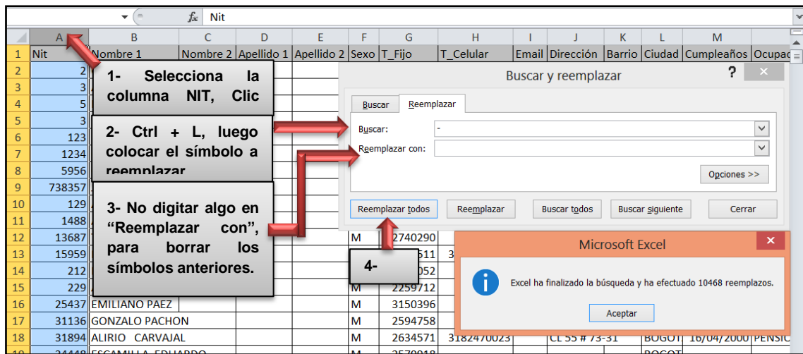
Figura 24. Herramienta reemplazar
